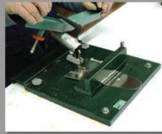
Test de flexion latérale du manche
