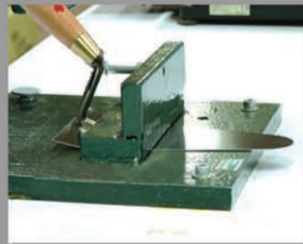
Test de flexion axiale du manche
