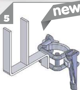
Support de plinthe protection périphérique
